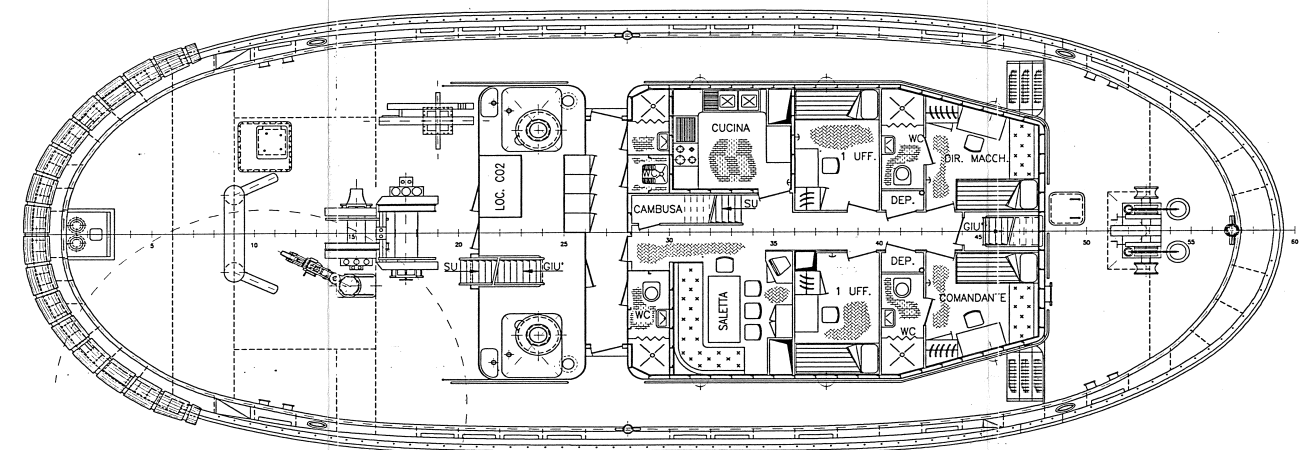
PONTE COPERTA
