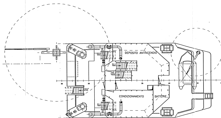
PONTE SUPERIORE
